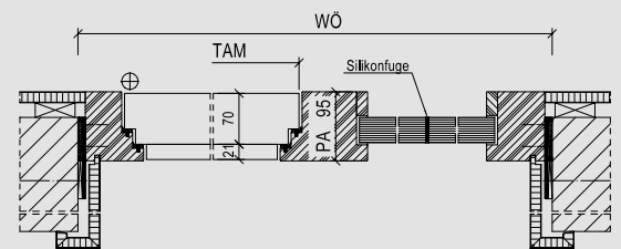
Detailzeichnung zu Bild 01
